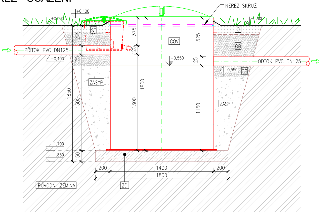
ŘEZ - OSAZENÍ
